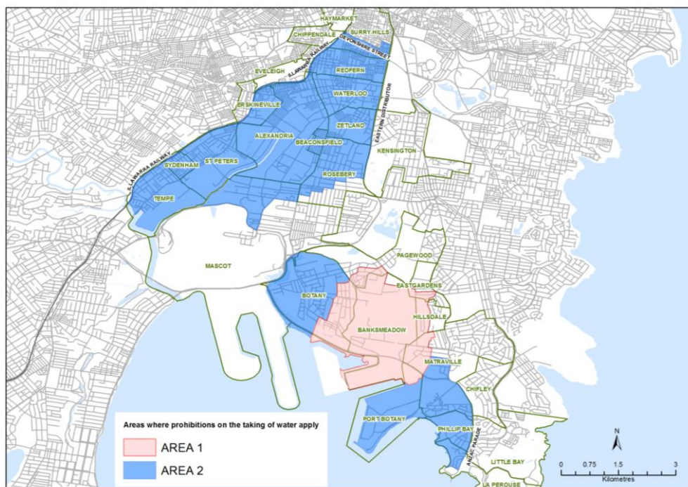
图 1. 限水令区域 1 区和 2 区
